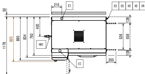
Planta
